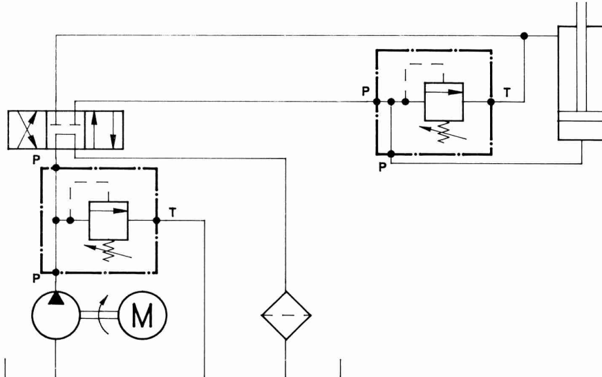
TİPİK DEVRE ÖRNEĞİ / TYPICAL CIRCUIT EXAMPLE
